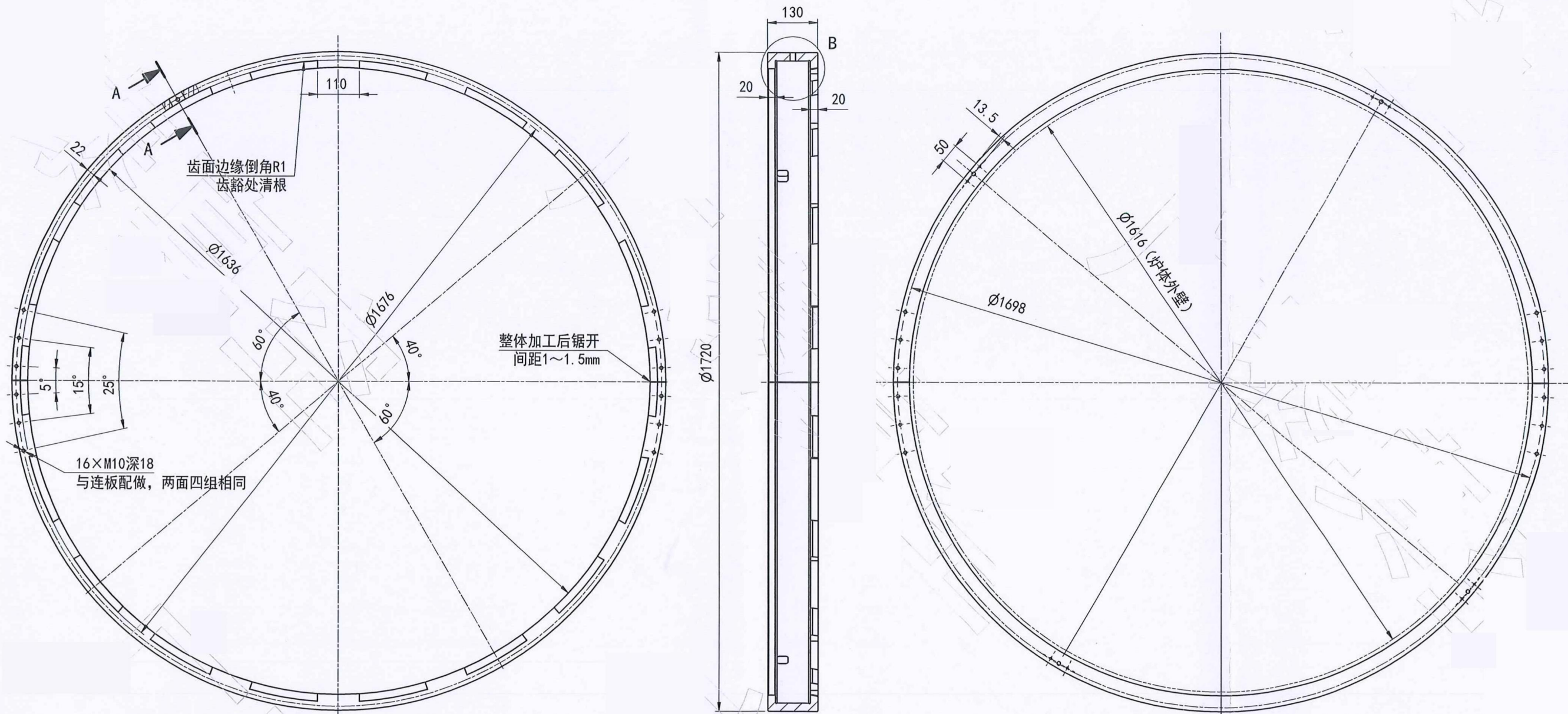
附件二：S2628加工图纸（图号：S01280.115-1）
